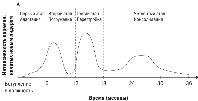
Рис. 4.1. Волны изменений
